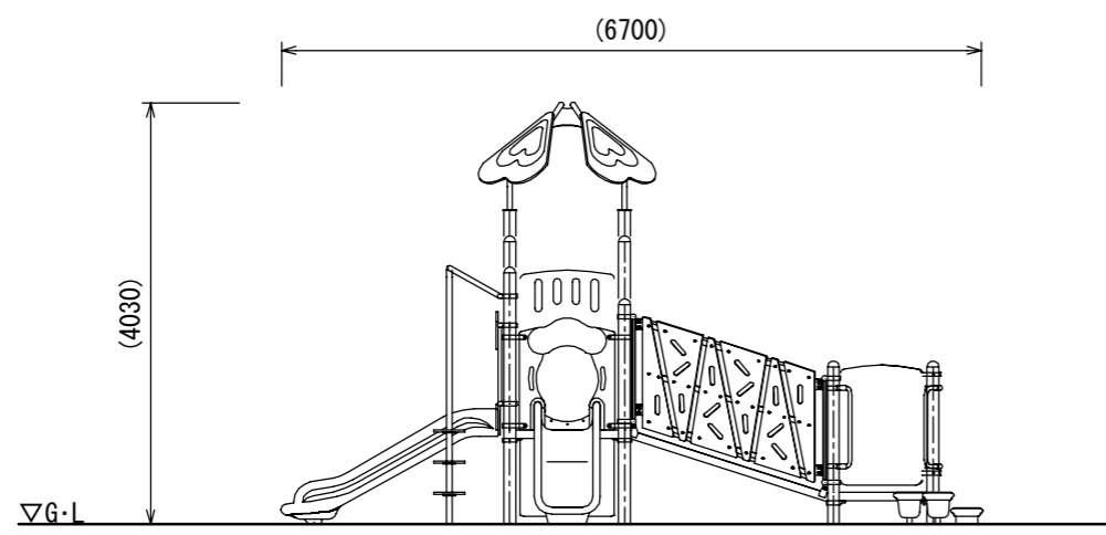
A立面図
