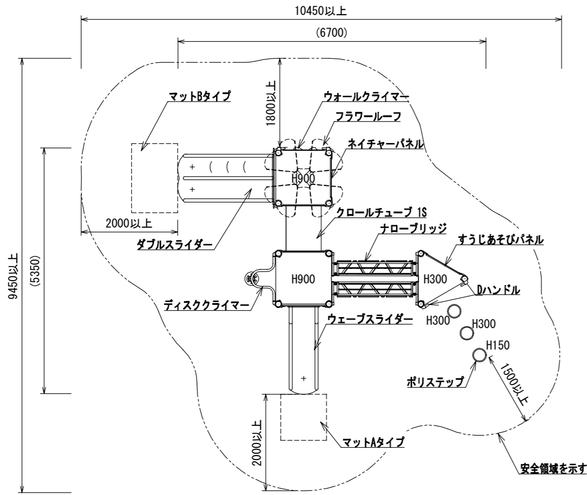
平面図
