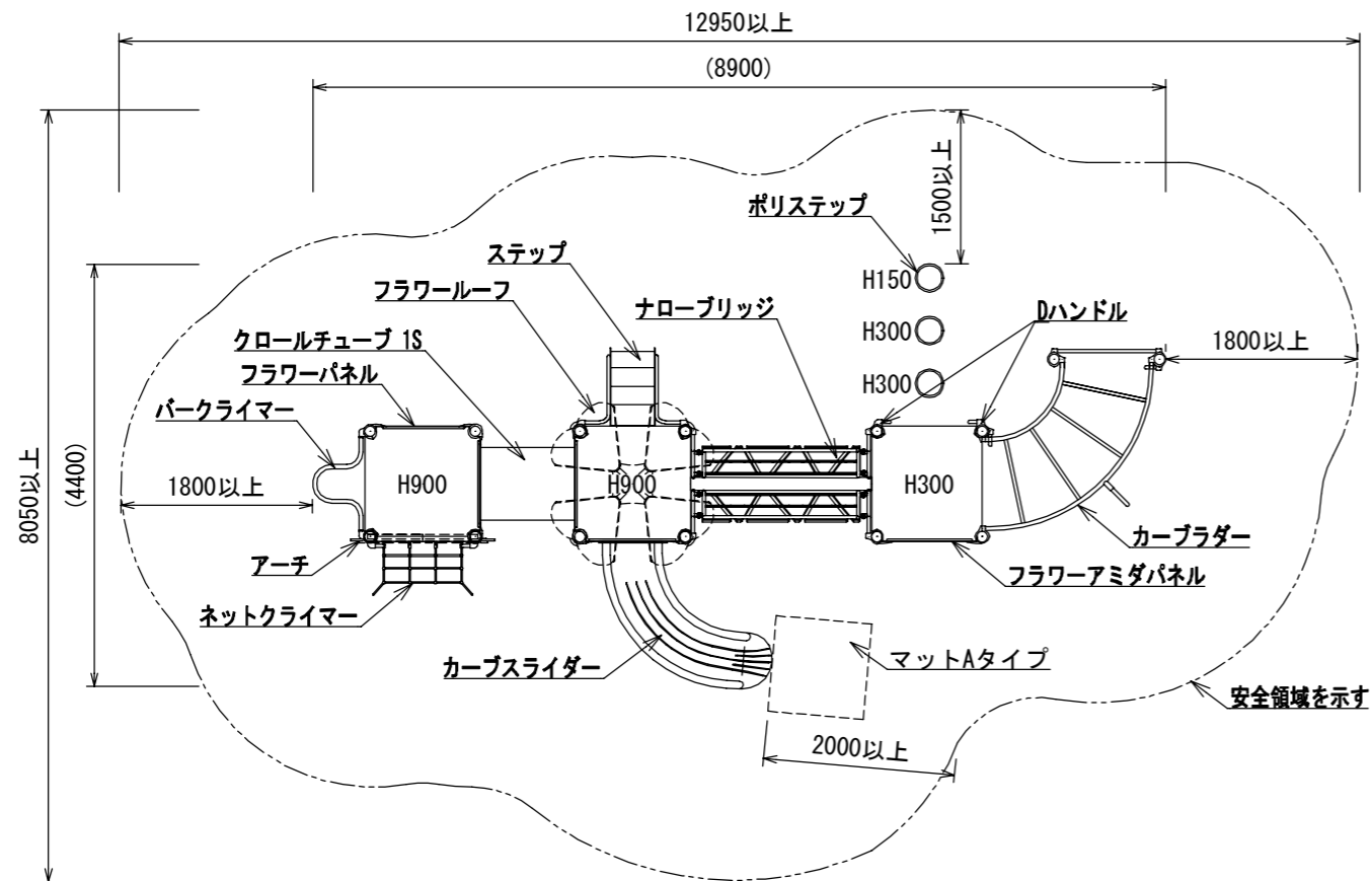
平面図
