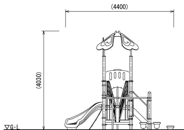
B立面図
