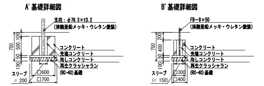
基礎詳細図 S=1:30 (A1) S=1:60 (A3)
