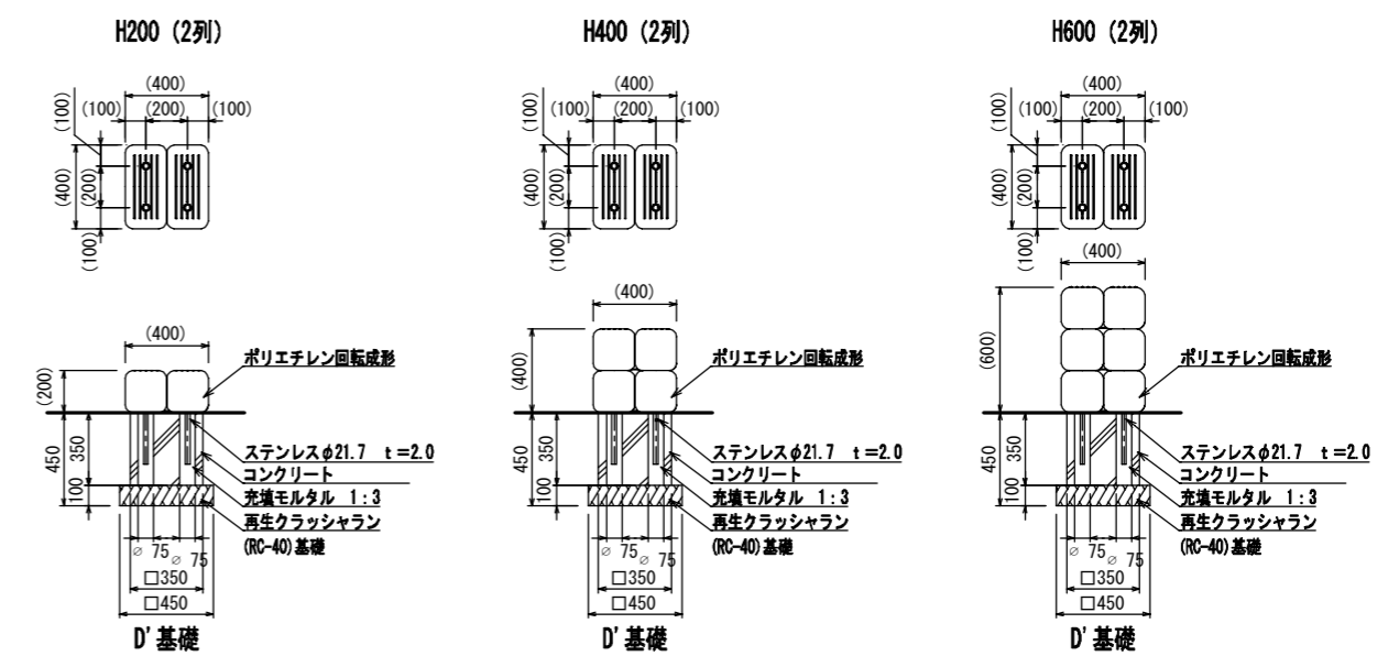
カラフルキャラメル詳細図 S=1:20 (A1) S=1:40 (A3)
