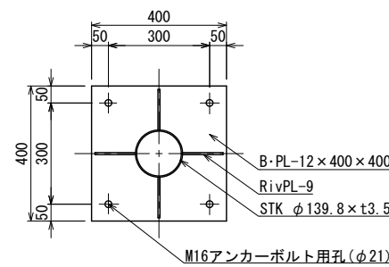
ベースプレート詳細図 S=1:10 (A3 S=1:20)
