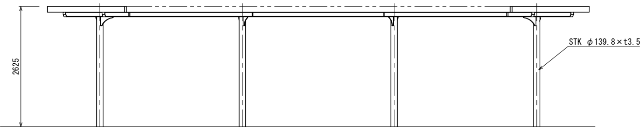
立面図
