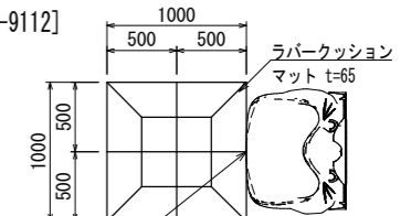
スライダー先端とマットの平面図 中央部の端を合わせる事。
