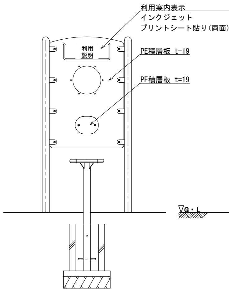
背面図
