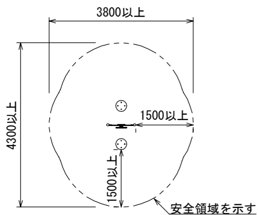
安全領域図 S=1:100
