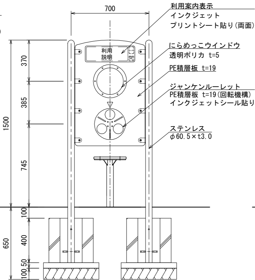
立面図
