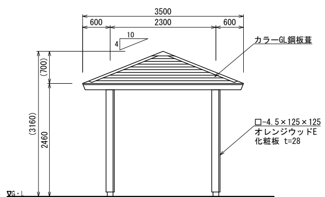
立面図
