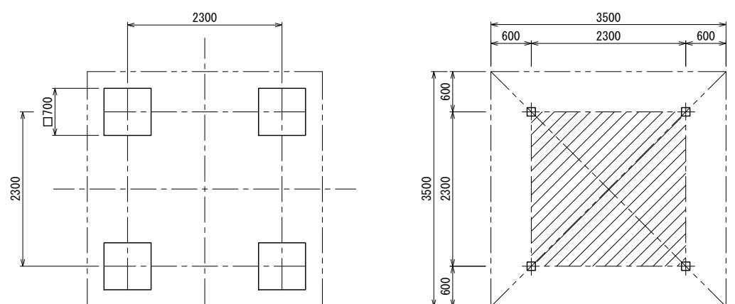
基礎伏図
