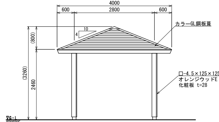
立面図
