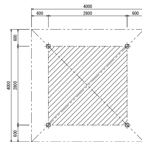
求積図
