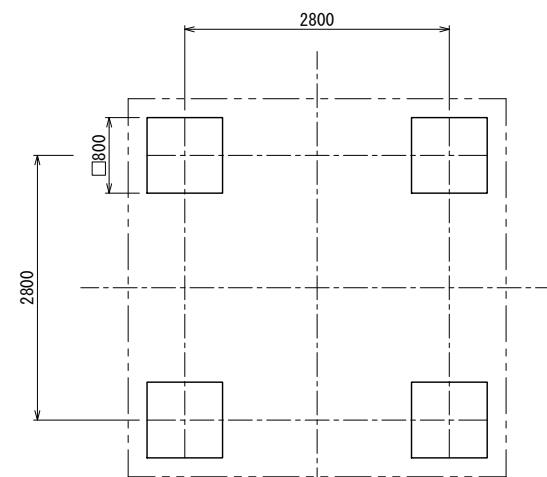
基礎伏図
