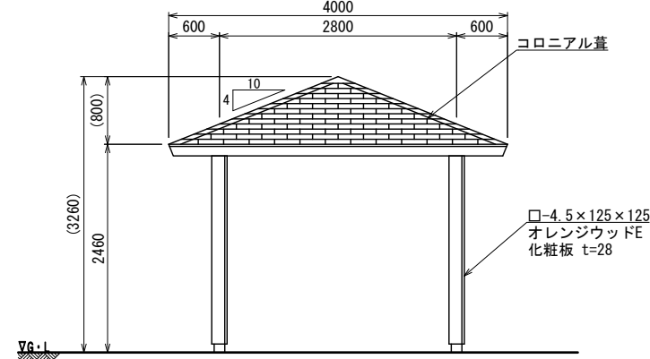
立面図
