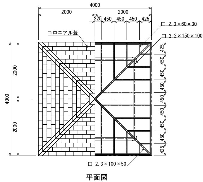
平面図
