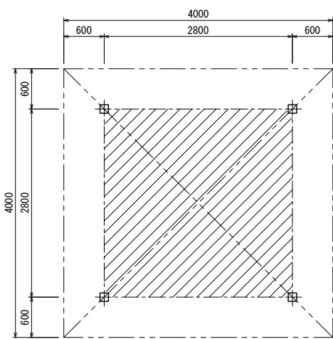
求積図
