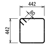
③ フープ筋: 4-D10
