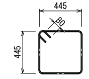
② フープ筋 (TOP): 2-D13
