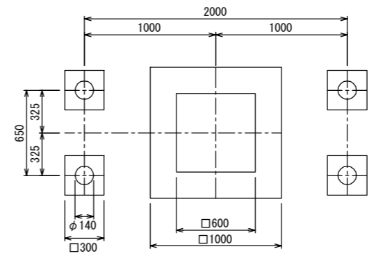
基礎伏せ図 S=1:20 (A3 S=1:40)
