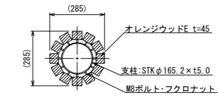
支柱断面図 S=1:10 (A3 S=1:20)
