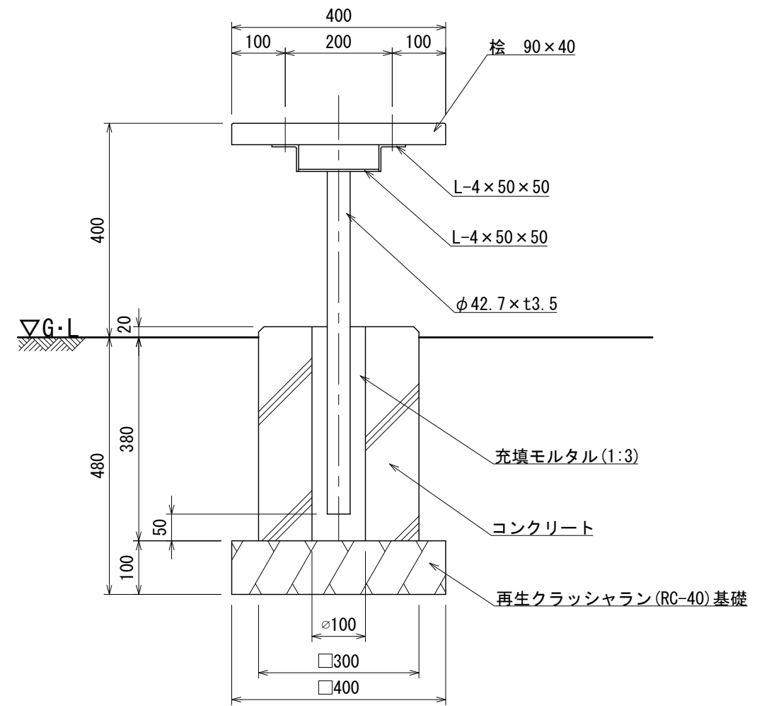
断面詳細図 S=1:10
