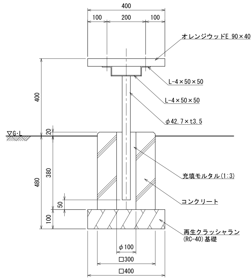
断面詳細図 S=1:10
