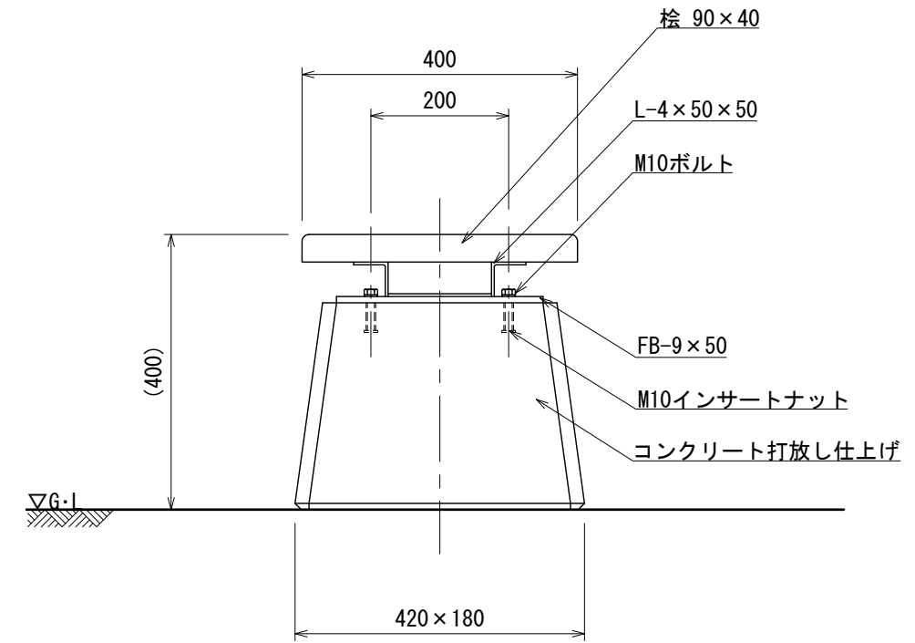
断面詳細図 S=1:10
