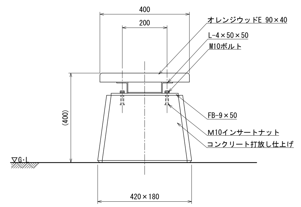
断面詳細図 S=1:10
