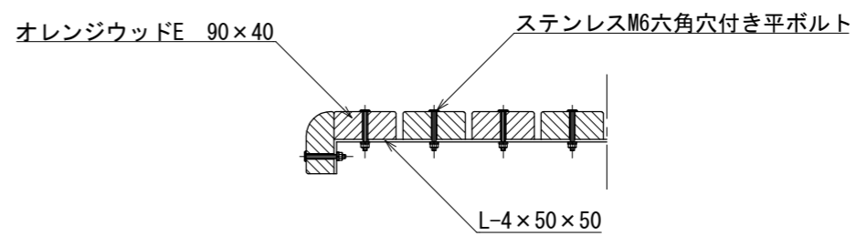
詳細図 S=1:10
