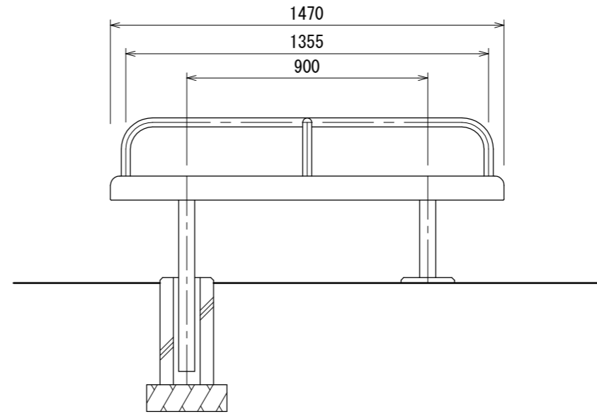
側面図
