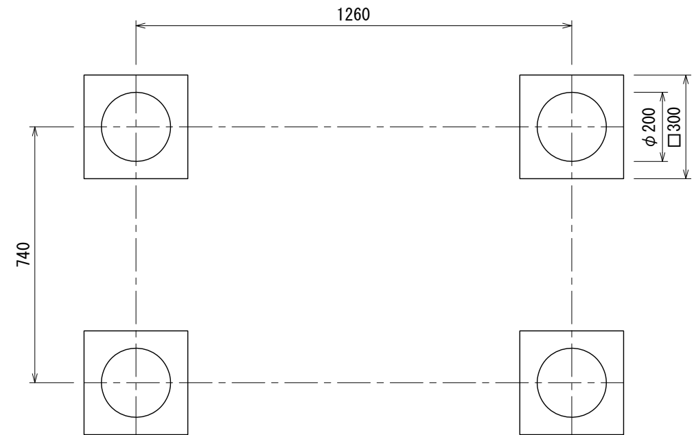
基礎伏図
