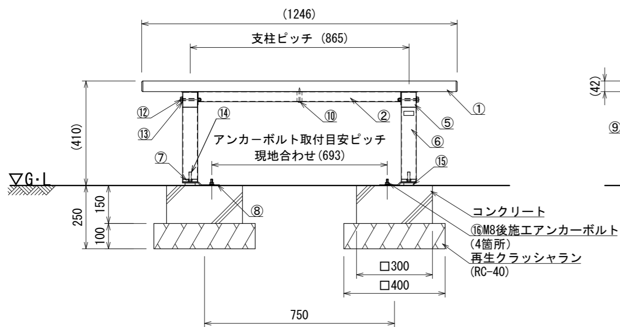
正面図
