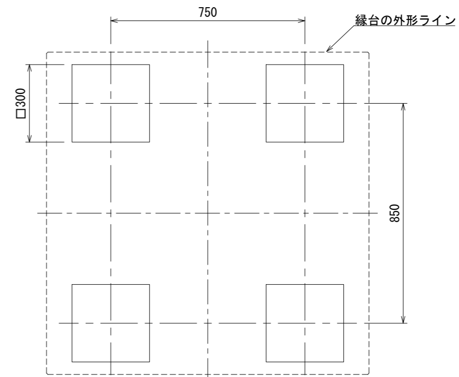
基礎伏図
