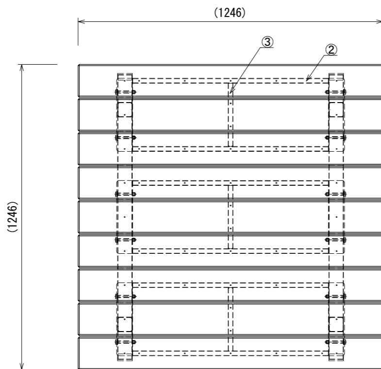
平面図
