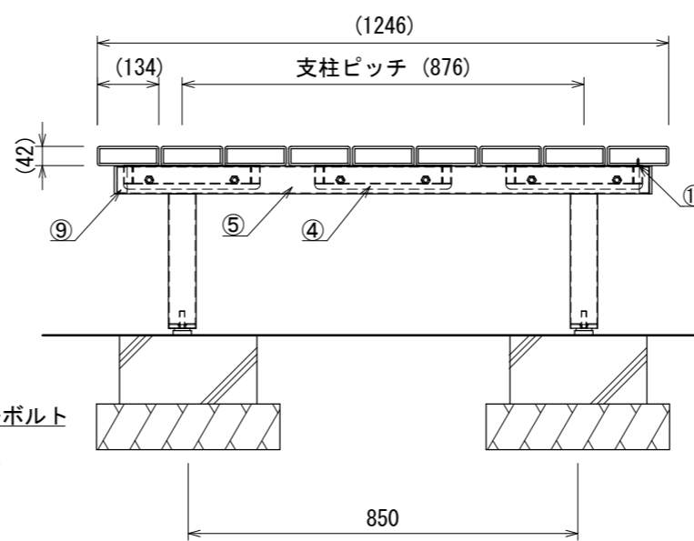
側面図
