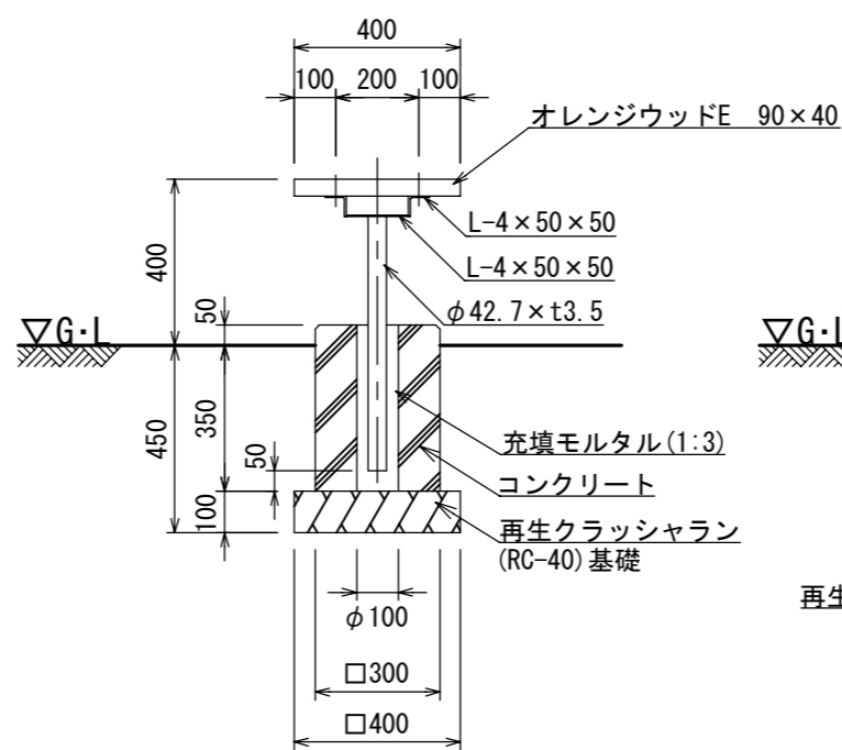
ベンチ詳細図 S=1:20
