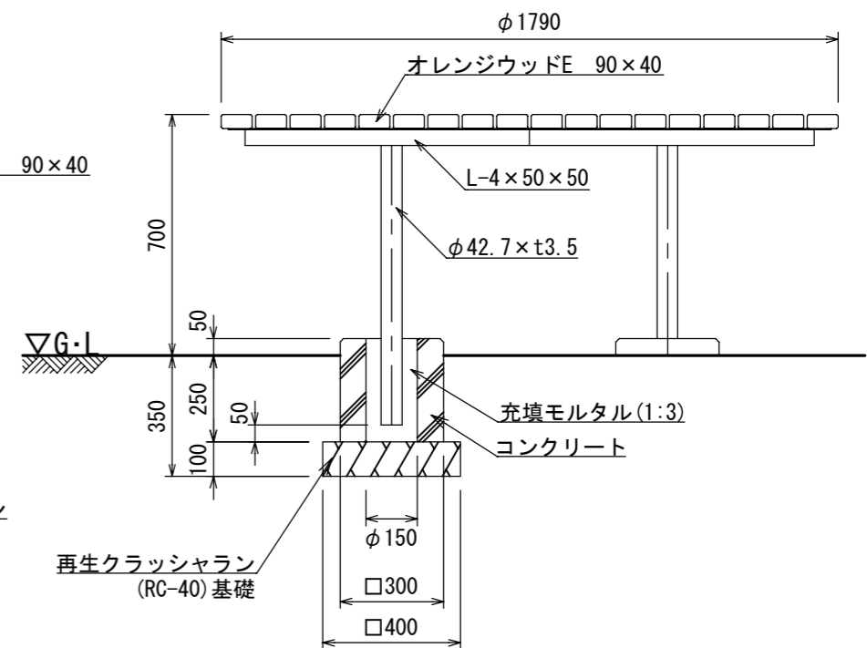
テーブル詳細図 S=1:20
