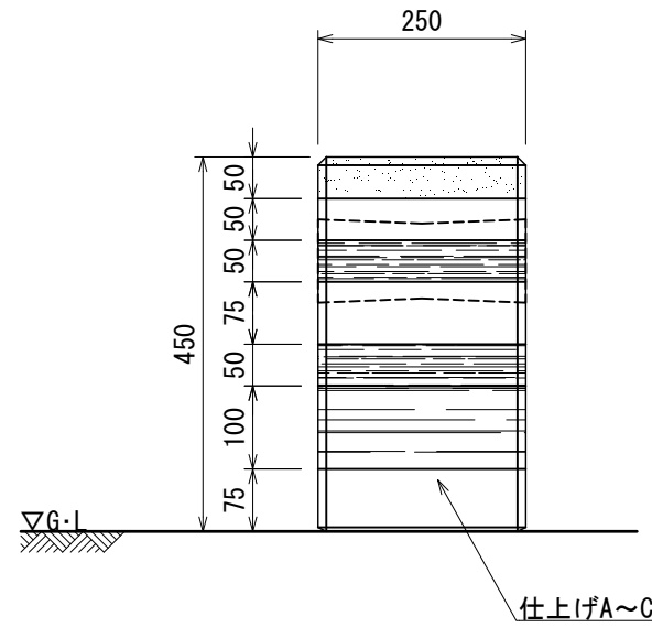
側面図
