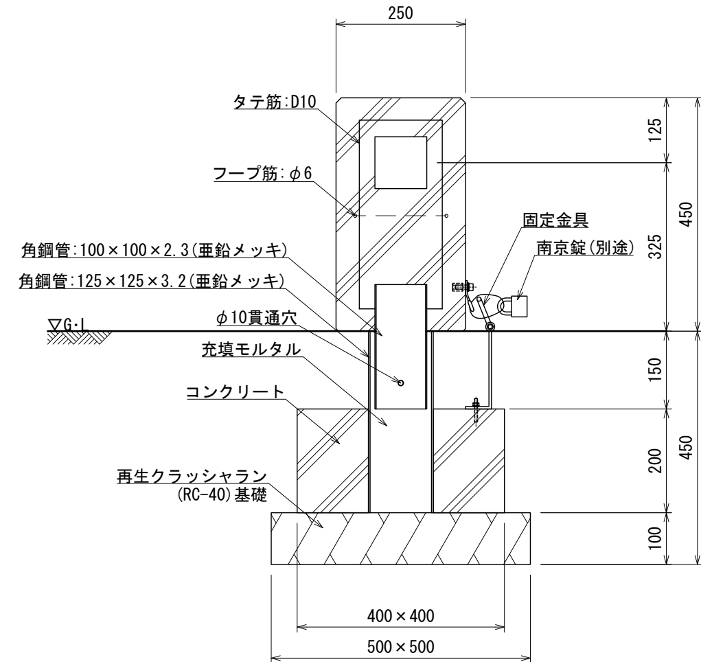
断面図
