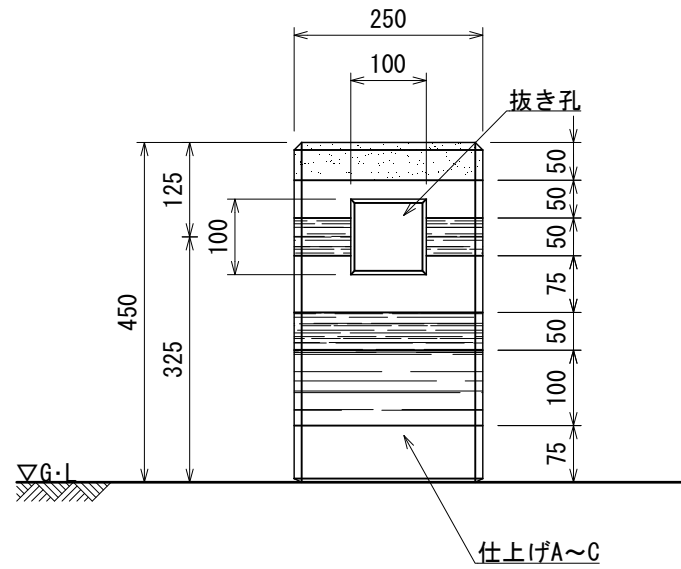
正面図
