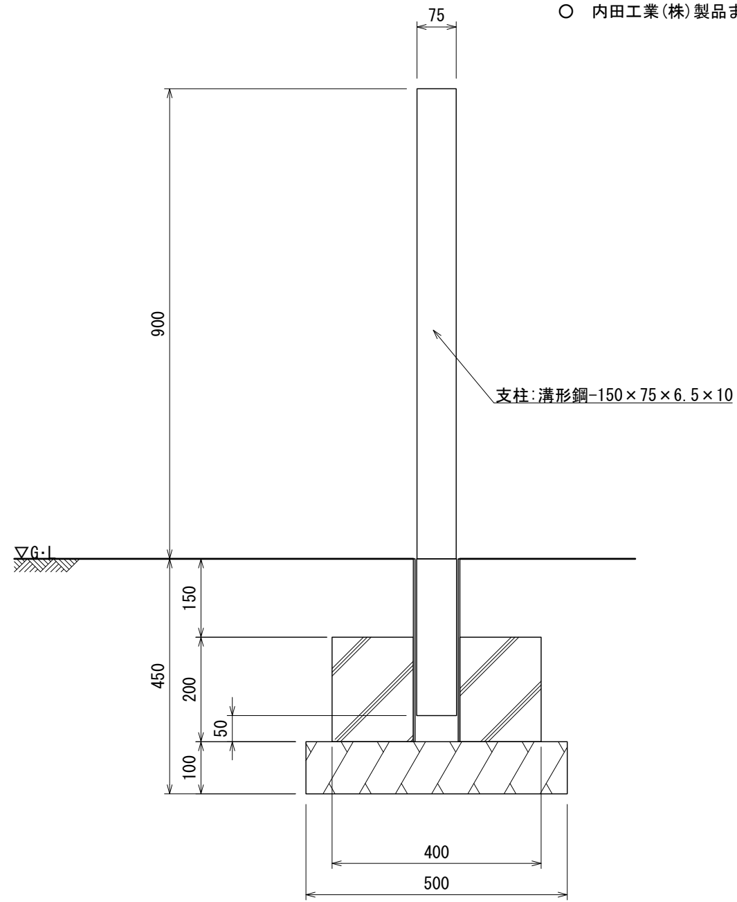
側面図
