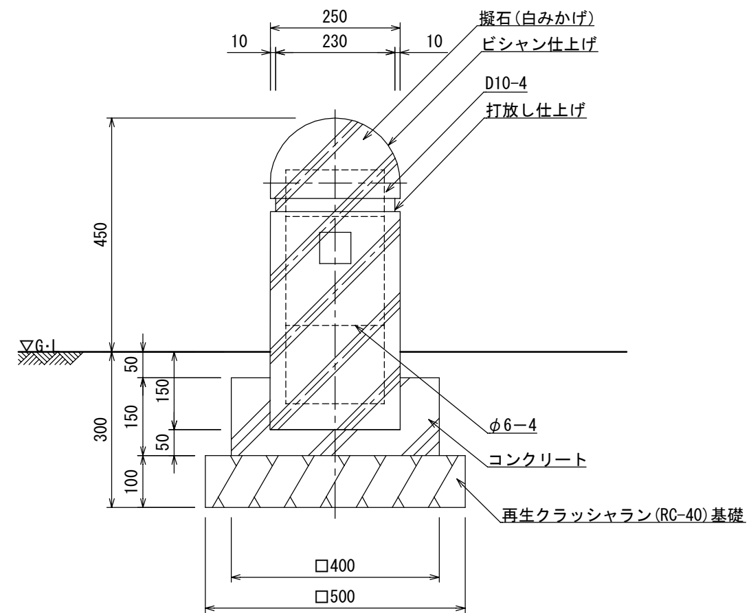
断面図
