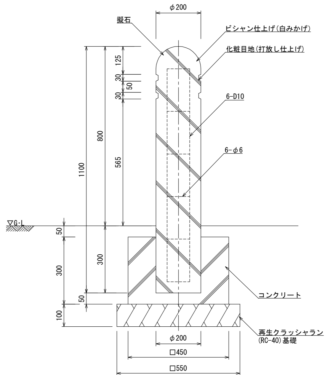
断面図
