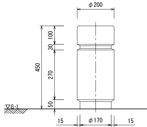
立面図
