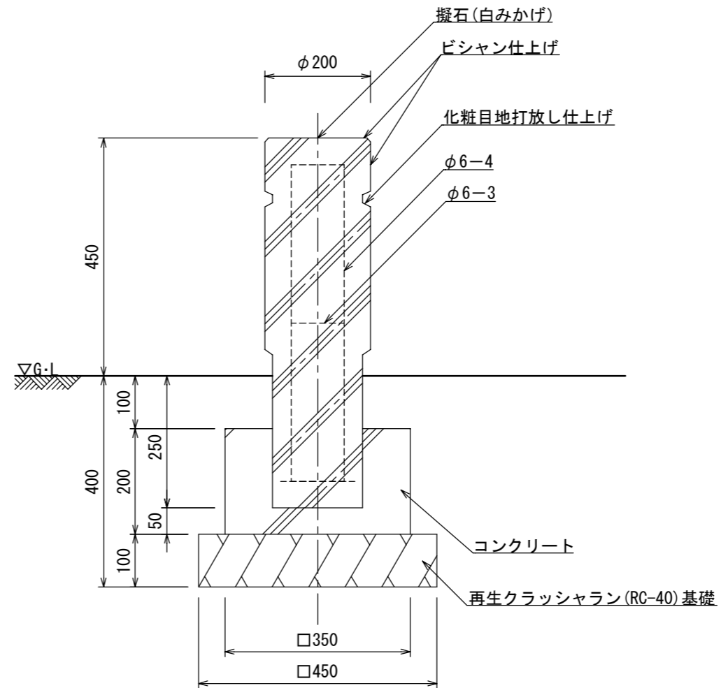
断面図
