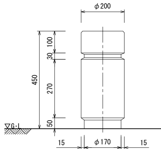
立面図
