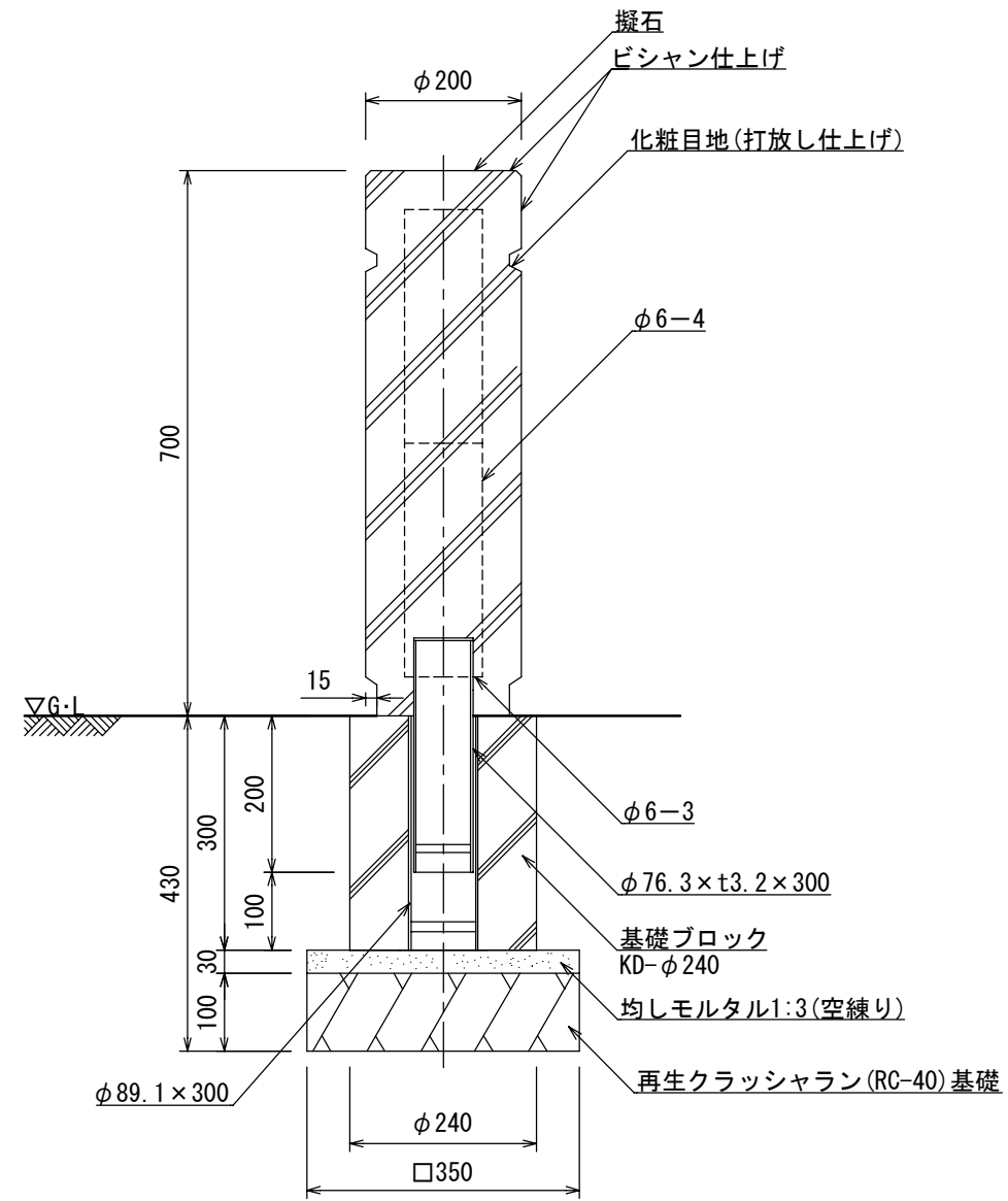
断面図
