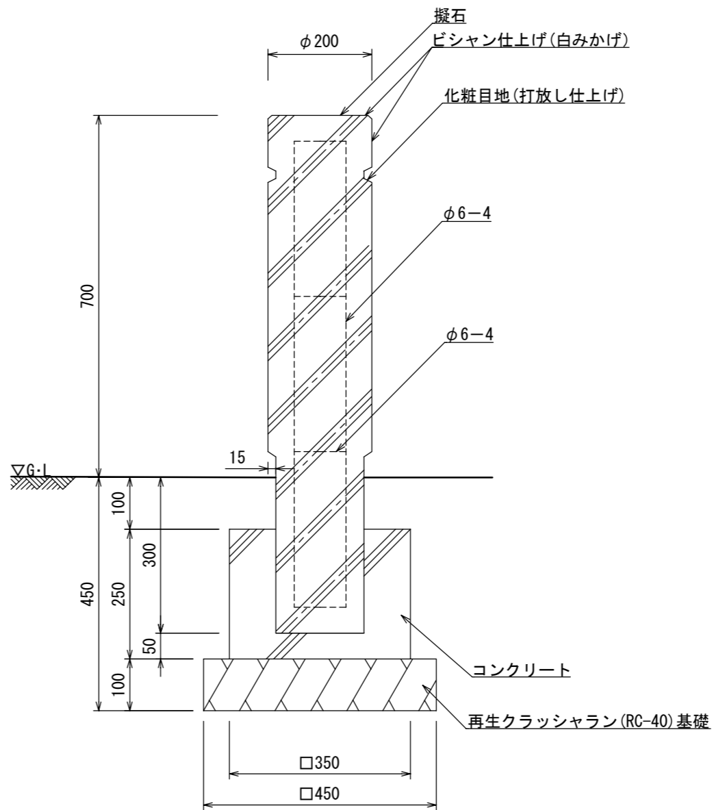
断面図
