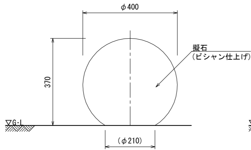
立面図
