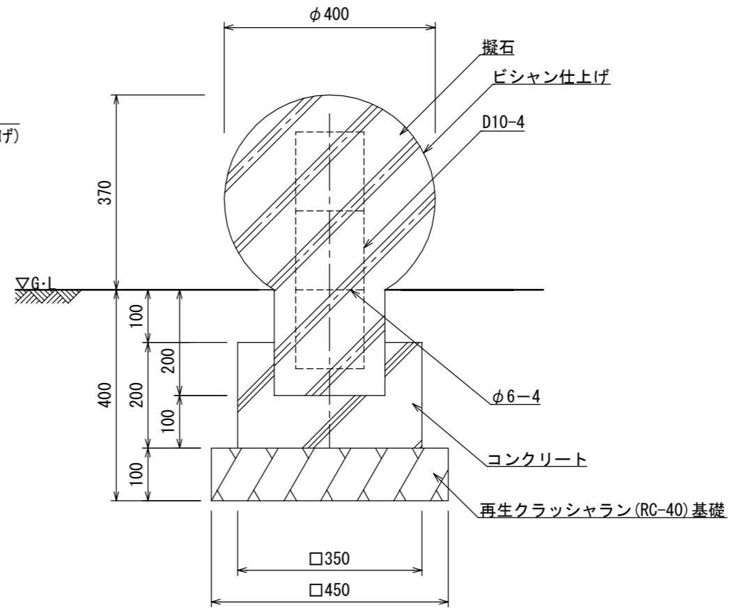
断面図
