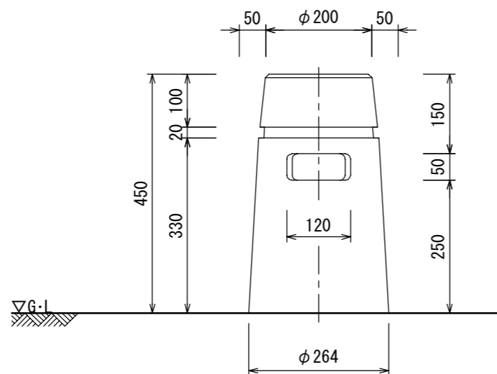
立面図
