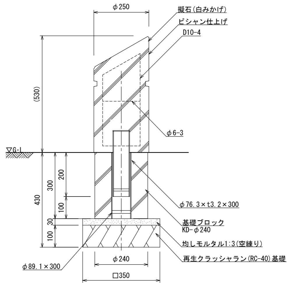
断面図
