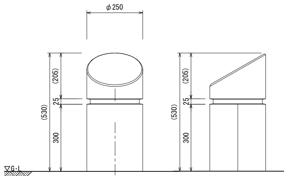
立面図
