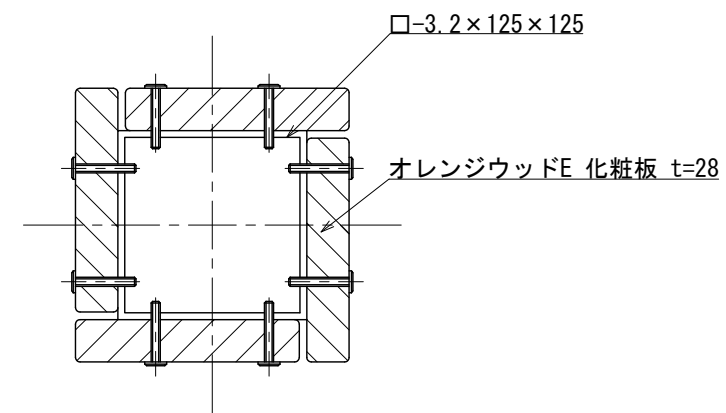
断面図 S=1:5
