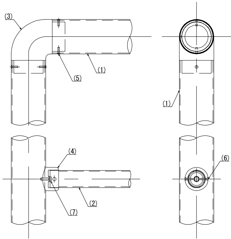
取付詳細図
