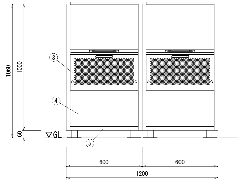
正面図
