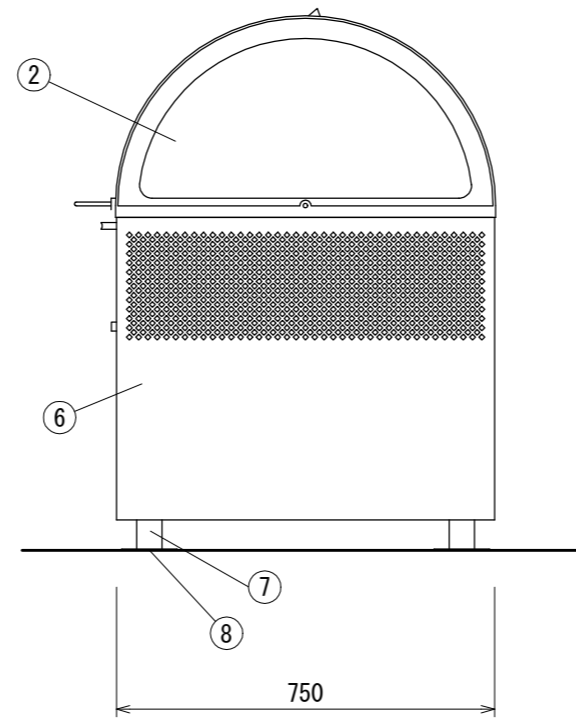
側面図
