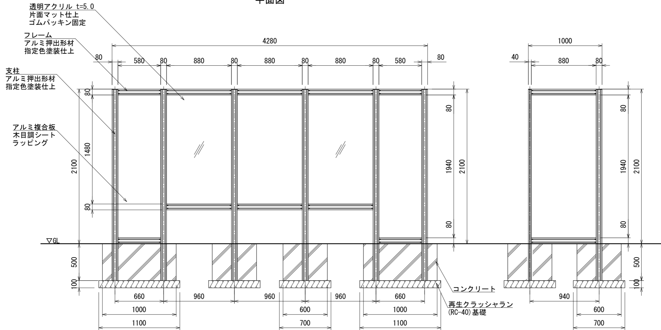
正面図
