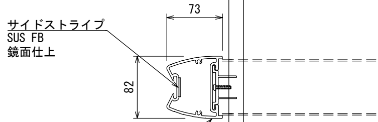
【平面図 S=1:5】
