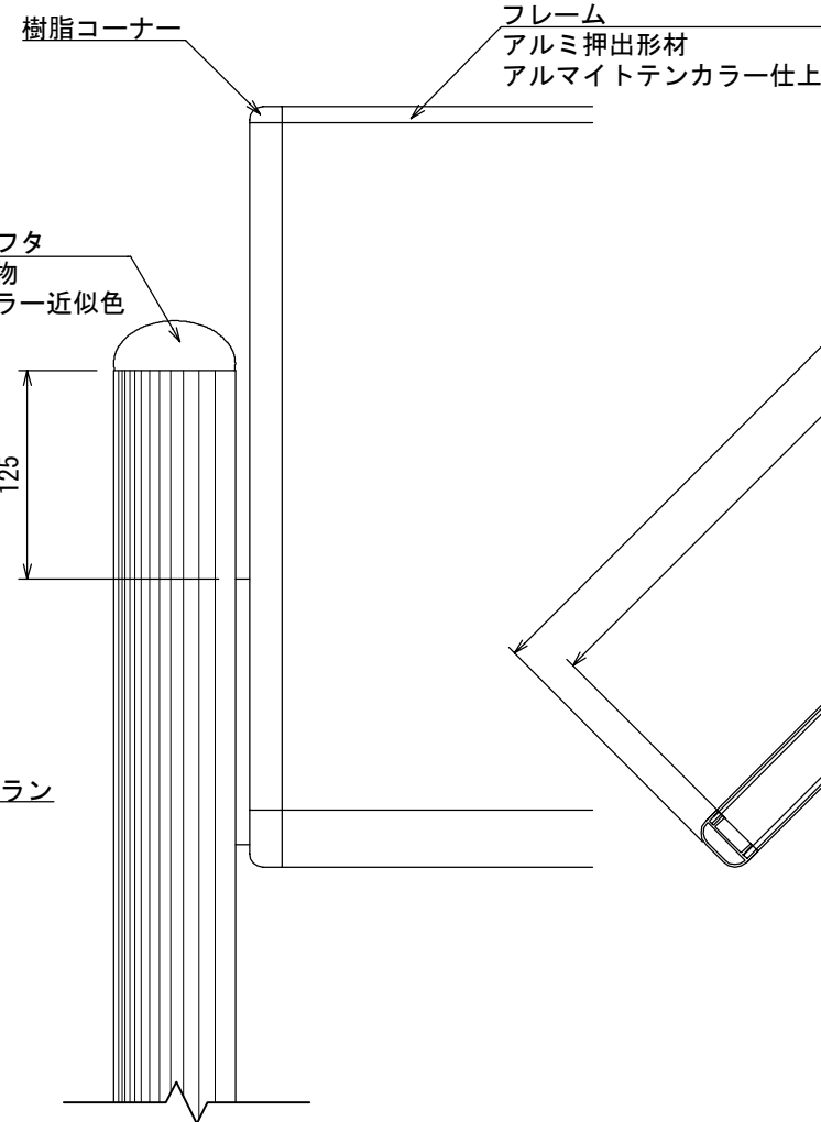
【正面図 S=1:5】
