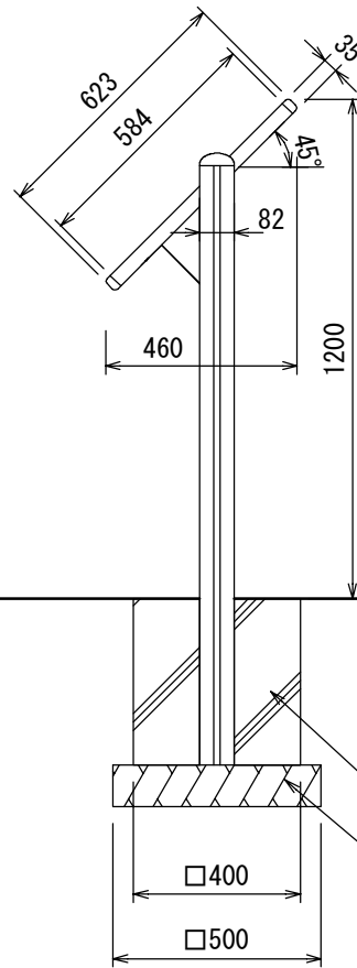
【側面図】
