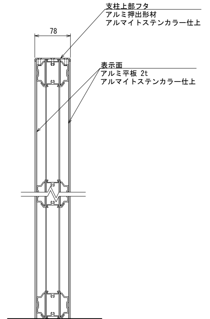
【側断面図 S=1:5】
