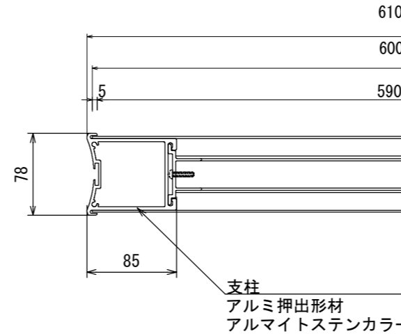
【平面図 S=1:5】
