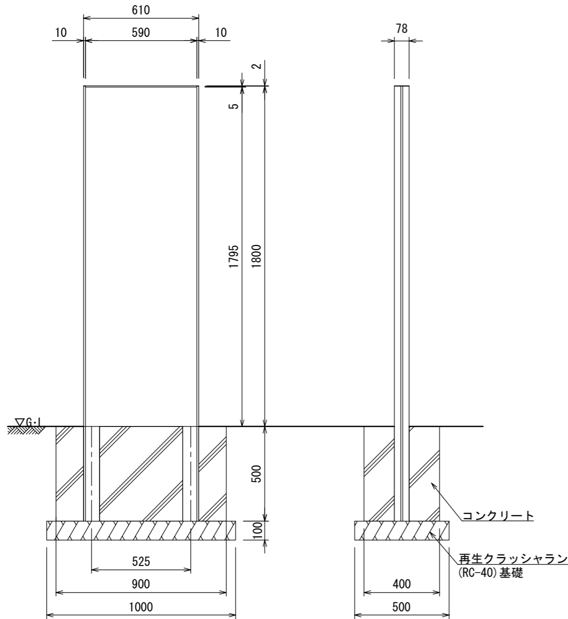
【正面図】
