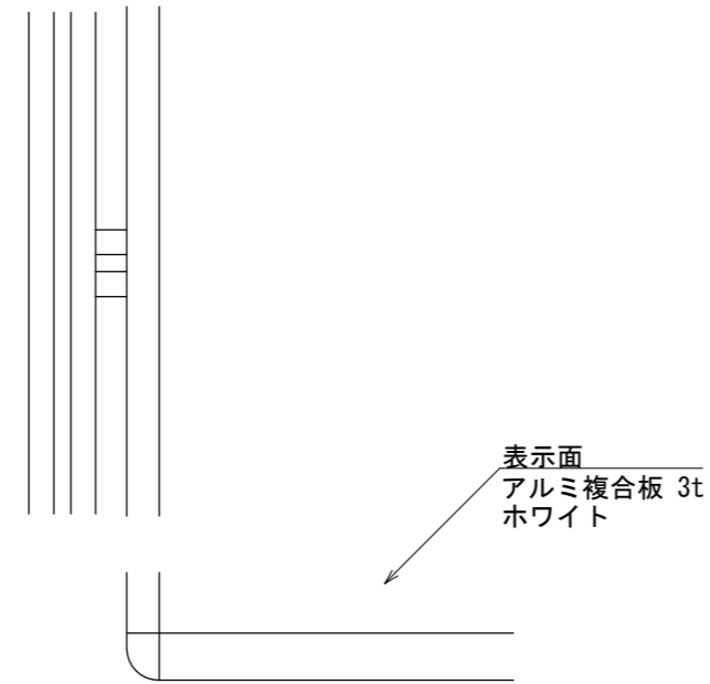
平面図 S=1:5
