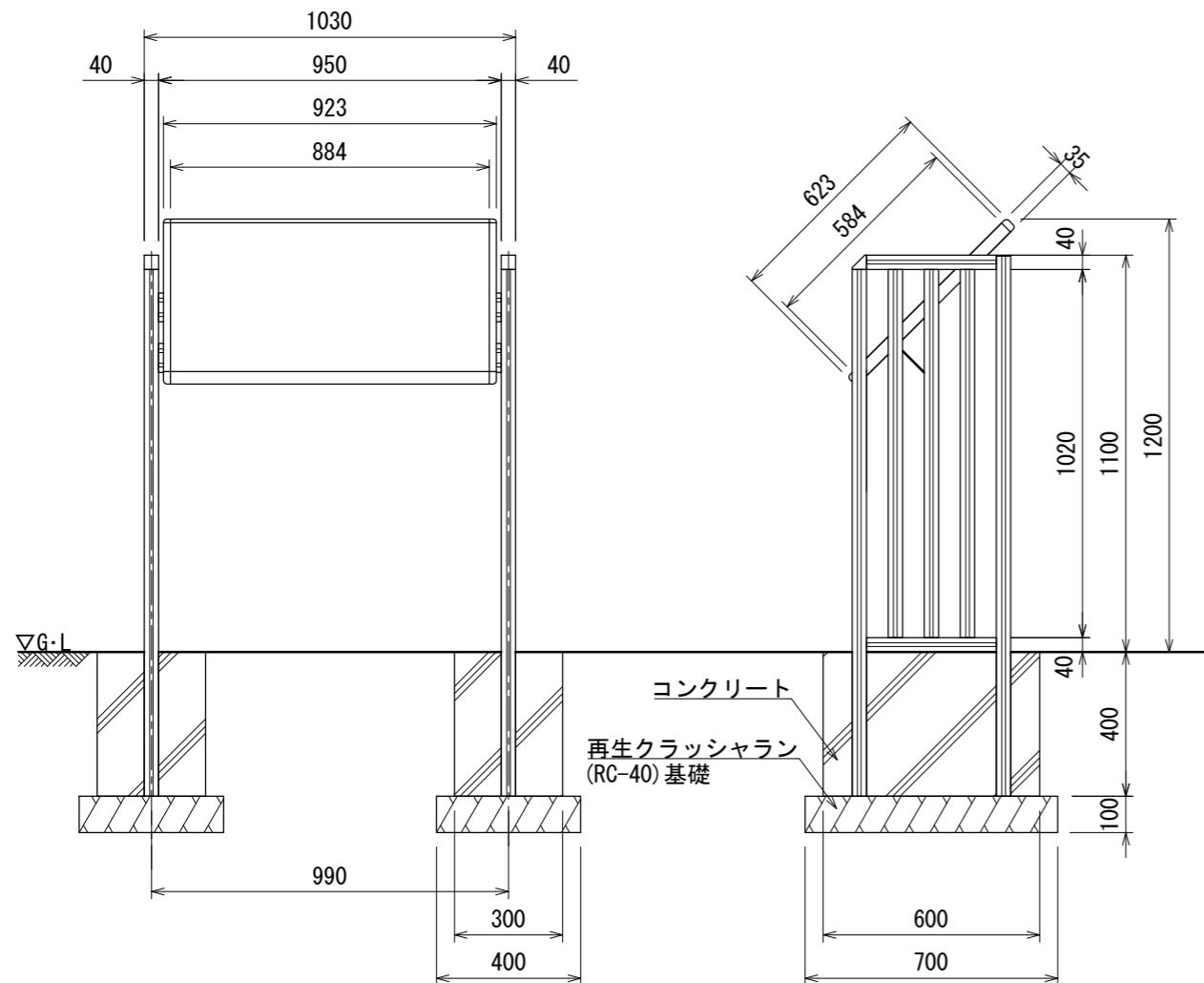
正面図
