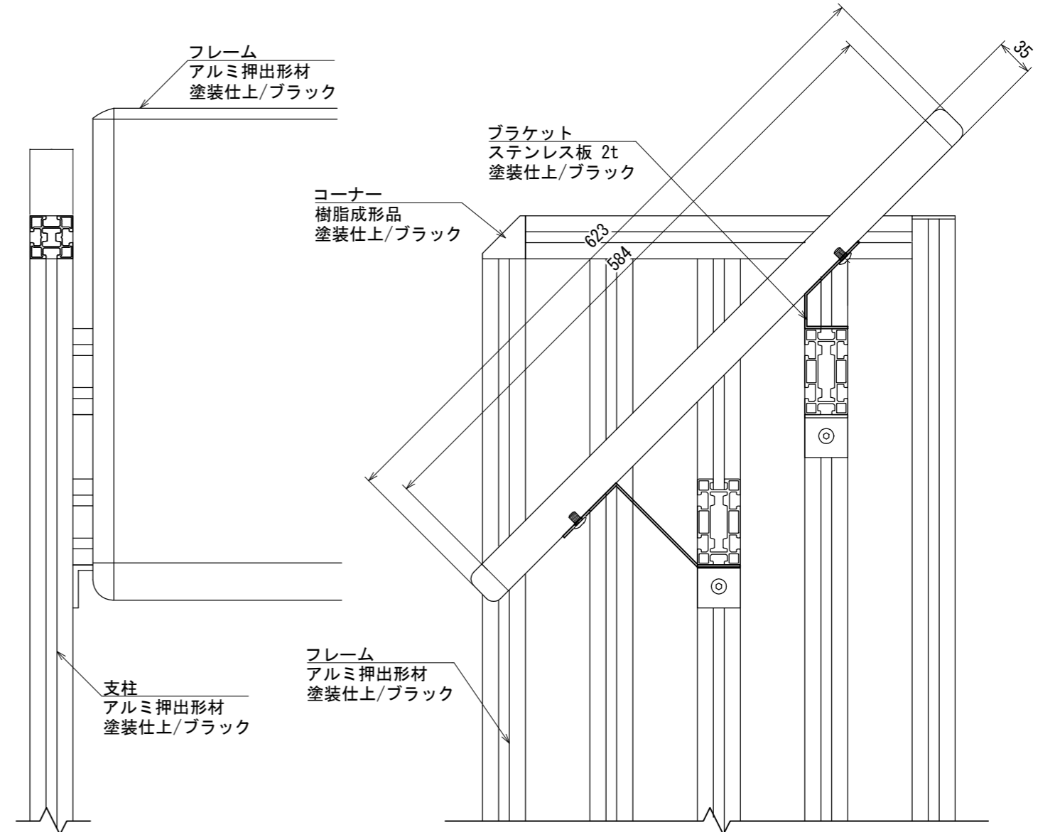
平面図 S=1:5
