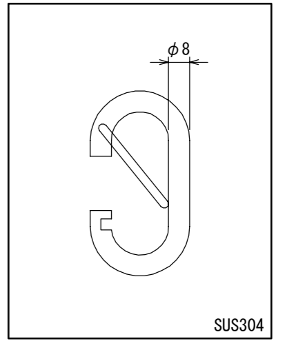
吊り下げフック (32個)
