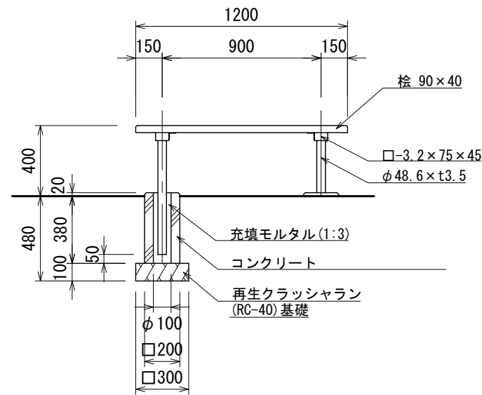
ベンチ部詳細図
