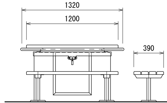
側面図
