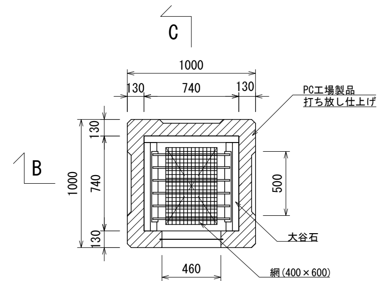
A断面図
