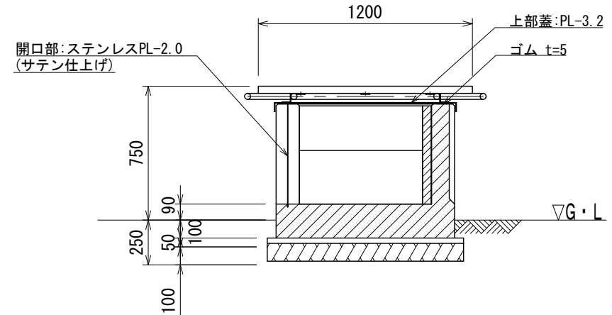
C断面図
