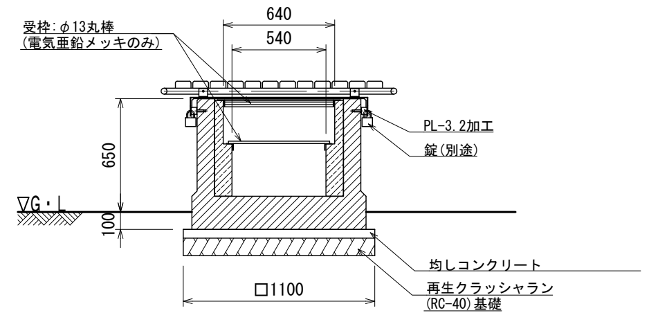
B断面図
