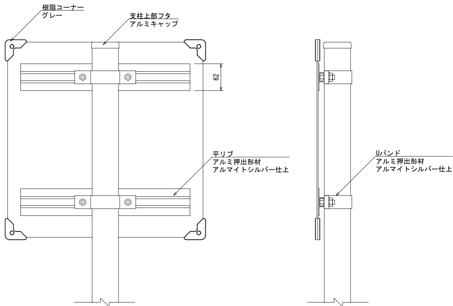
【背面図 S=1:5】
