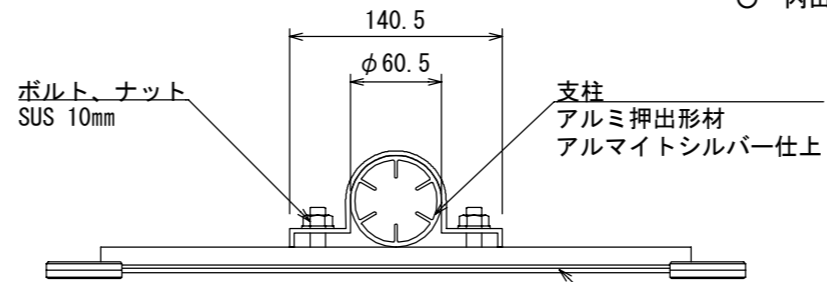
【平面図 S=1:5】
