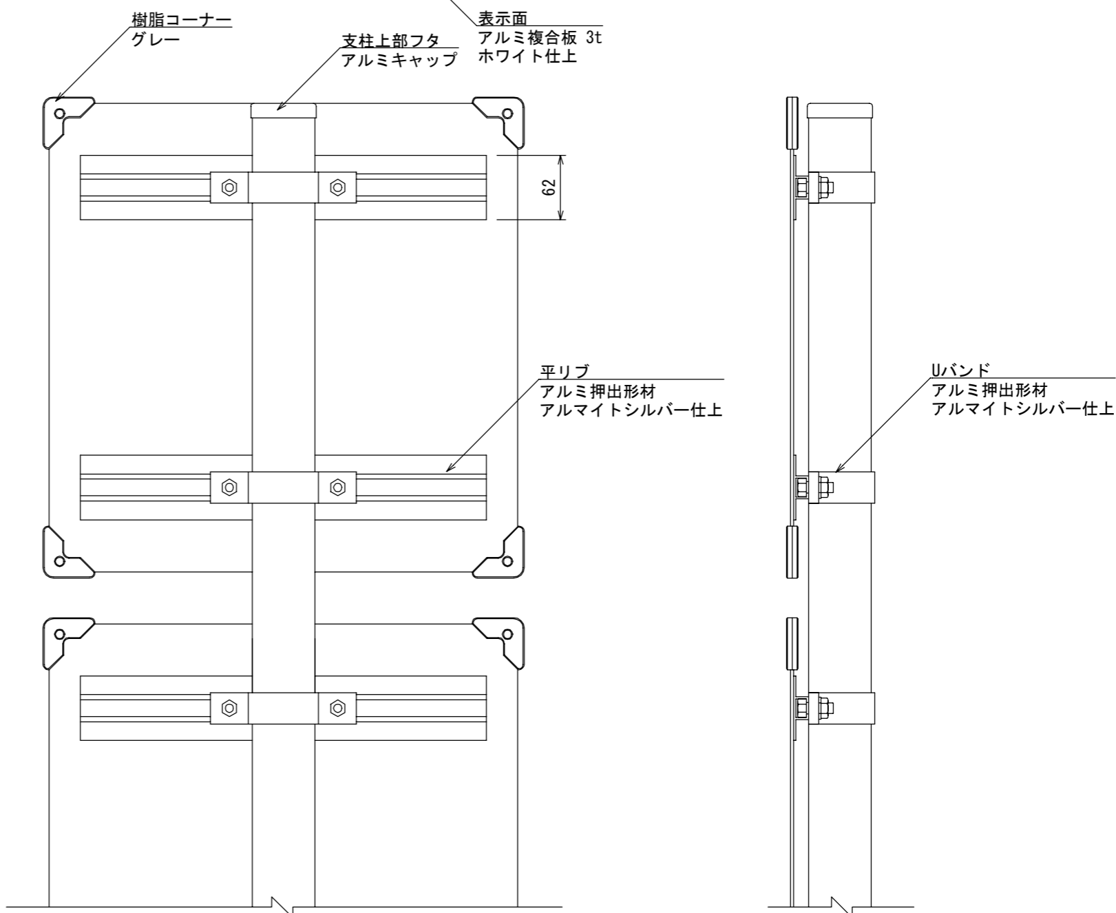
【背面図 S=1:5】
