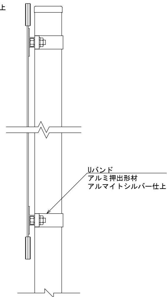
【側面図 S=1:5】
