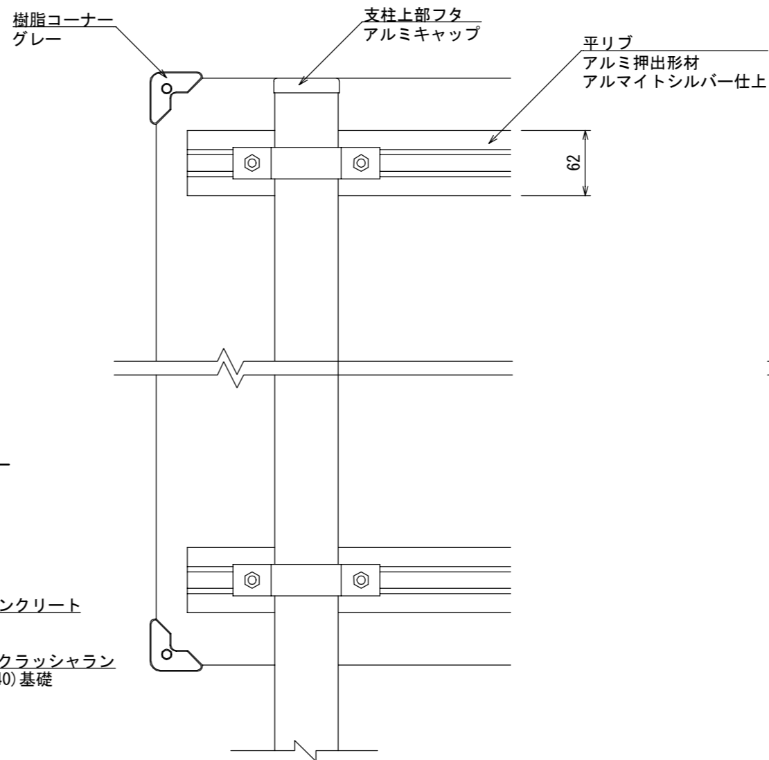
【背面図 S=1:5】
