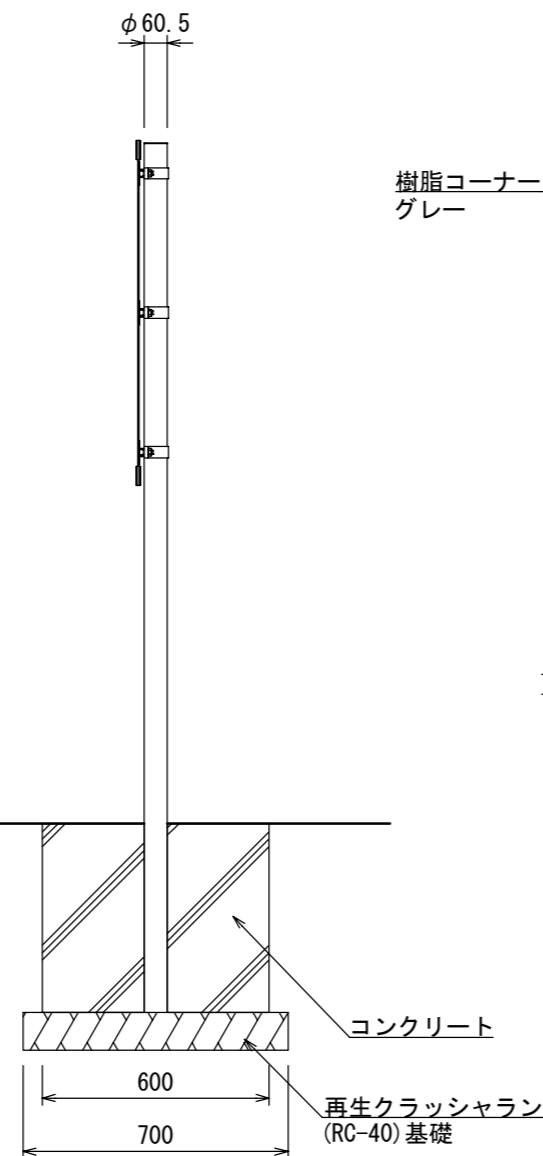
【側面図】
