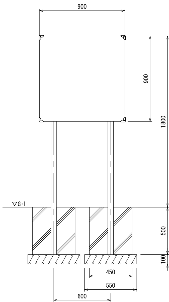
【正面図】
