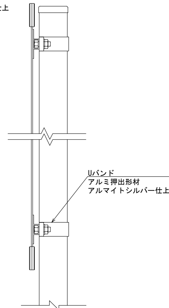
【側面図 S=1:5】
