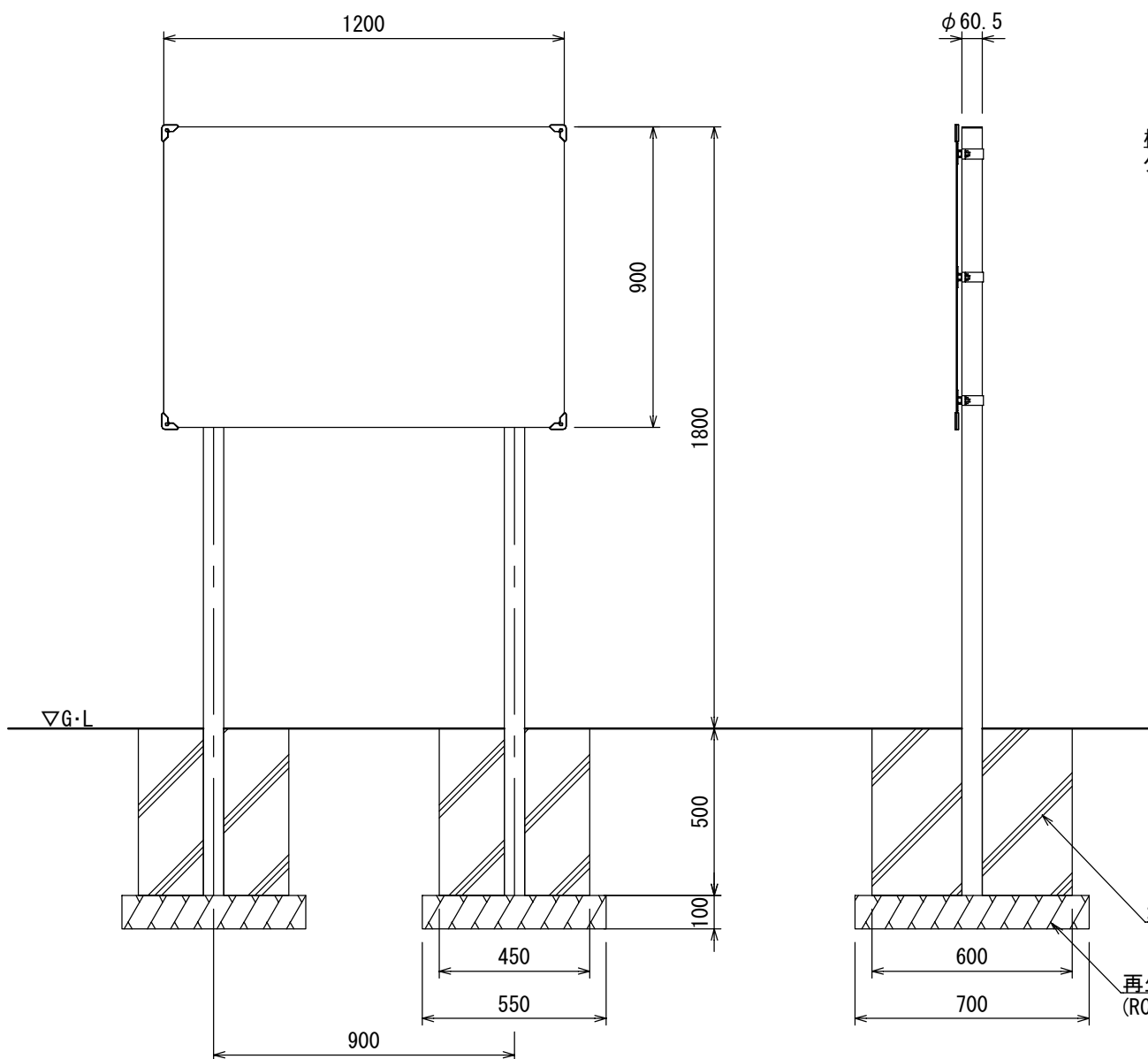
【正面図】
