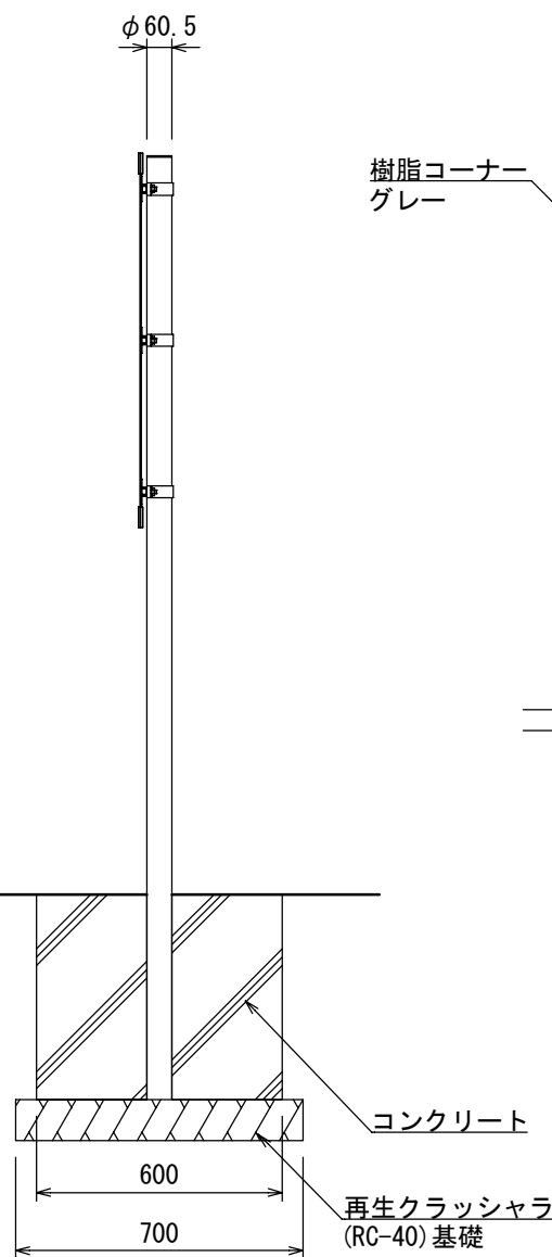
【側面図】
