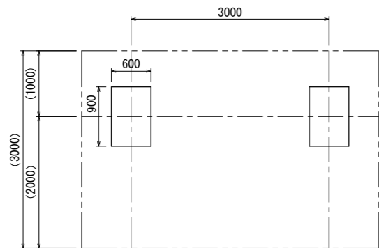
基礎伏図
