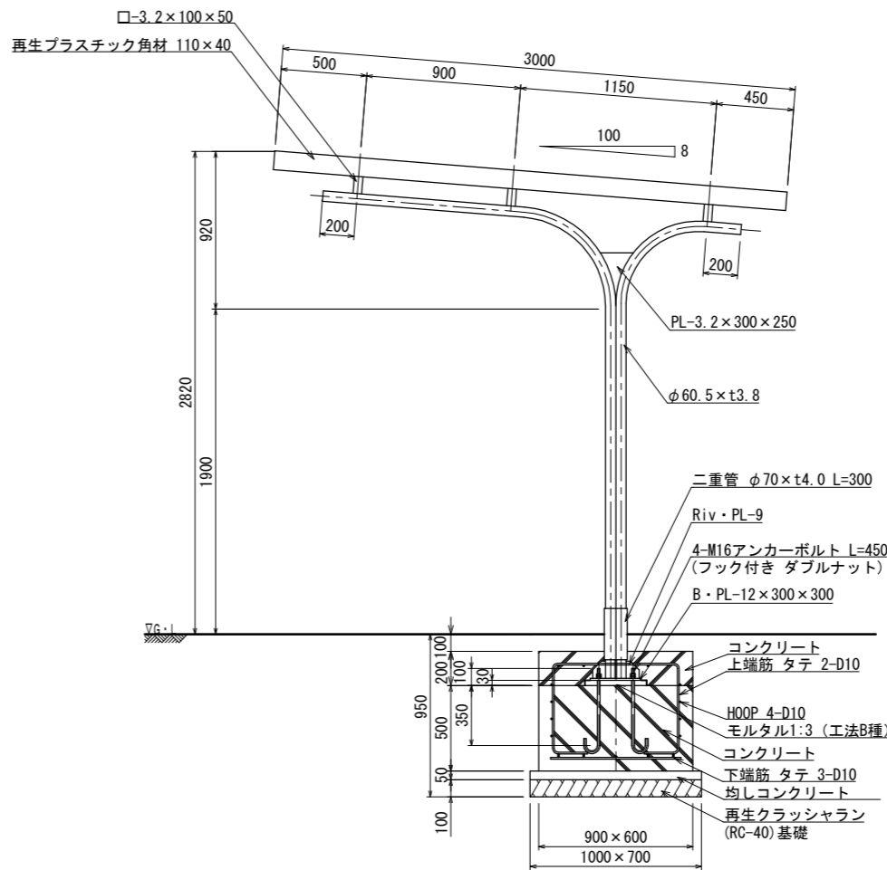
詳細図 S=1:20 (A3 S=1:40)
