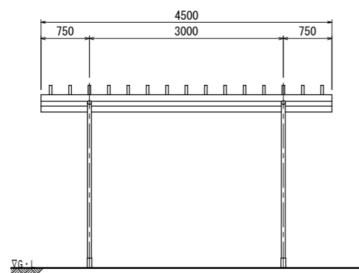
立面図
