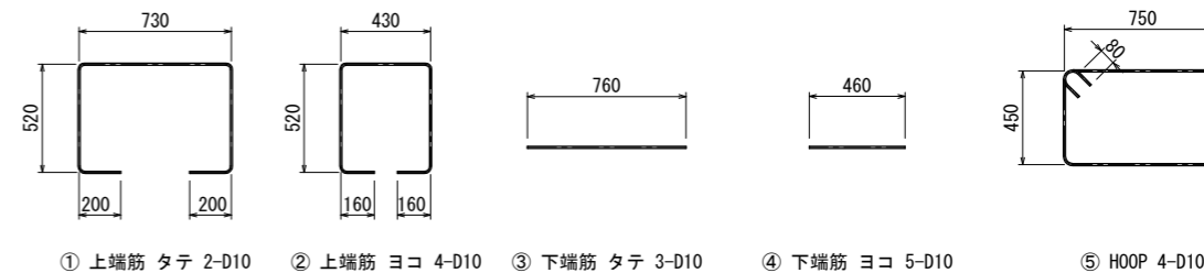
鉄筋図 S=1:20 (A3 S=1:40)
