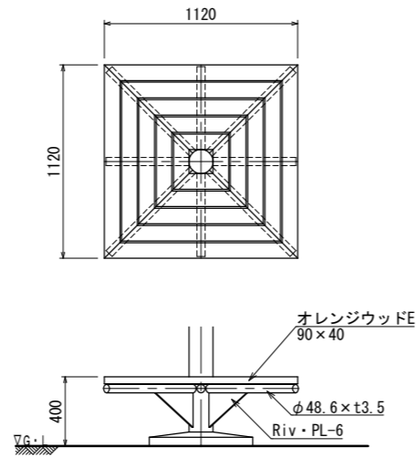
ベンチ詳細図 S=1:20 (A3 S=1:40)
