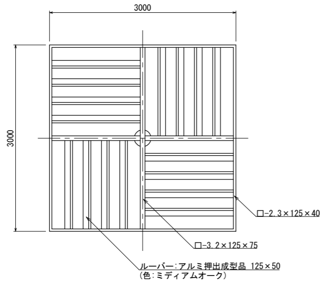
屋根伏図
