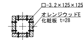
支柱断面図 S=1:10 (A3 S=1:20)
