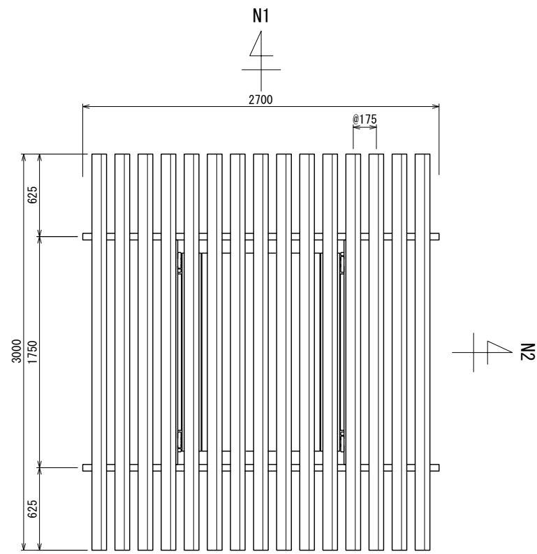
平面図 (※N1, N2は設置推奨方向)
