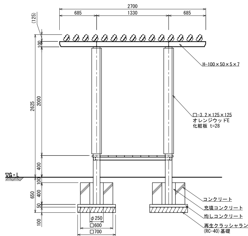
立面図
