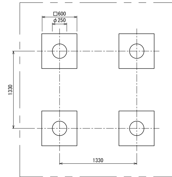
基礎伏図
