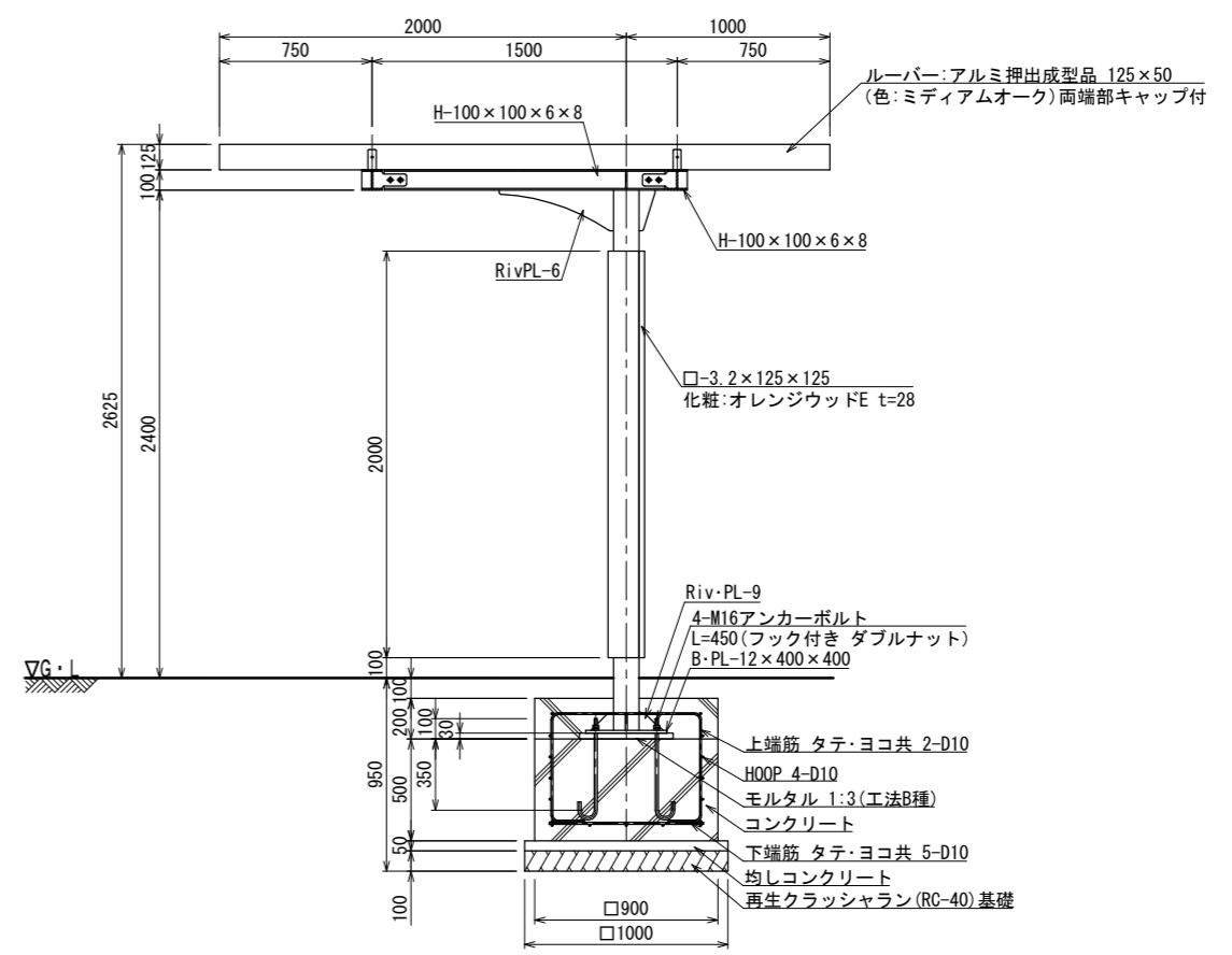
断面詳細図 S=1:20 (A3 S=1:40) 鉄筋加工図 S=1:20 (A3 S=1:40)
