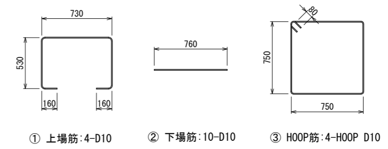
断面詳細図 S=1:20 (A3 S=1:40) 鉄筋加工図 S=1:20 (A3 S=1:40)
