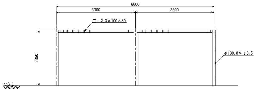
立面図
