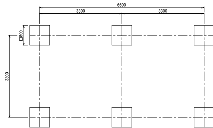
基礎伏図
