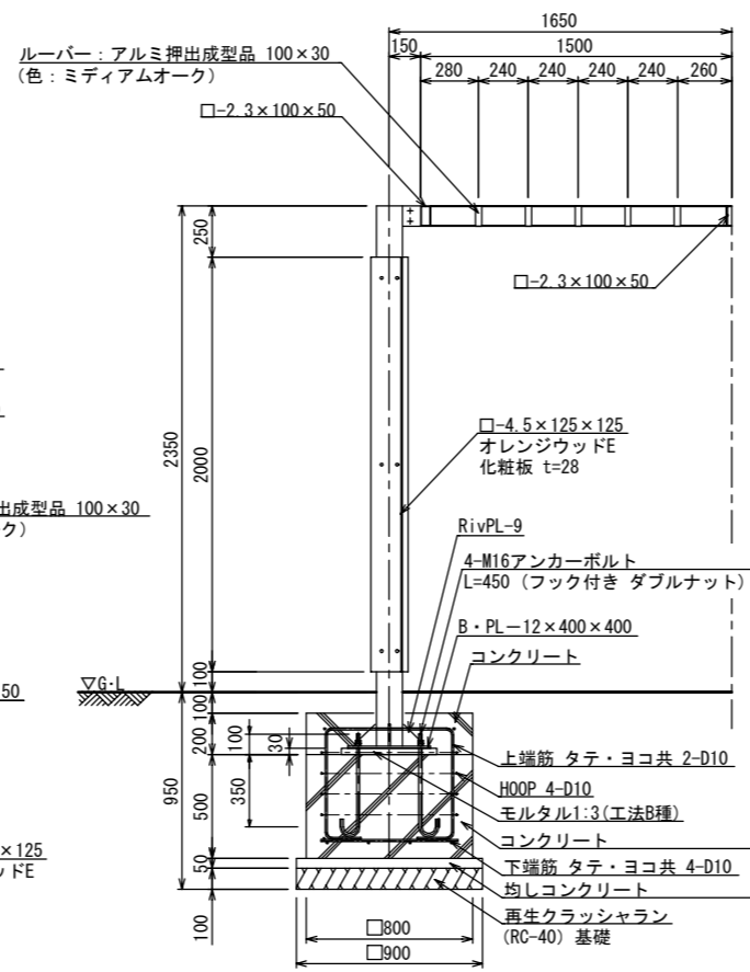
断面詳細図 S=1:20 (A3 S=1:40)
