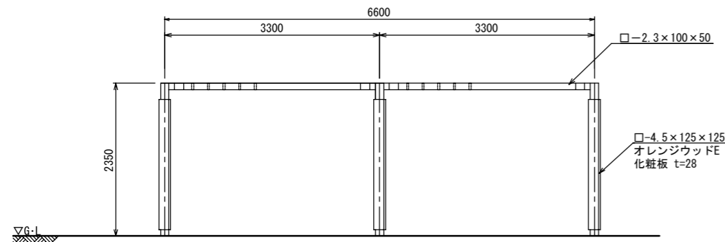
立面図
