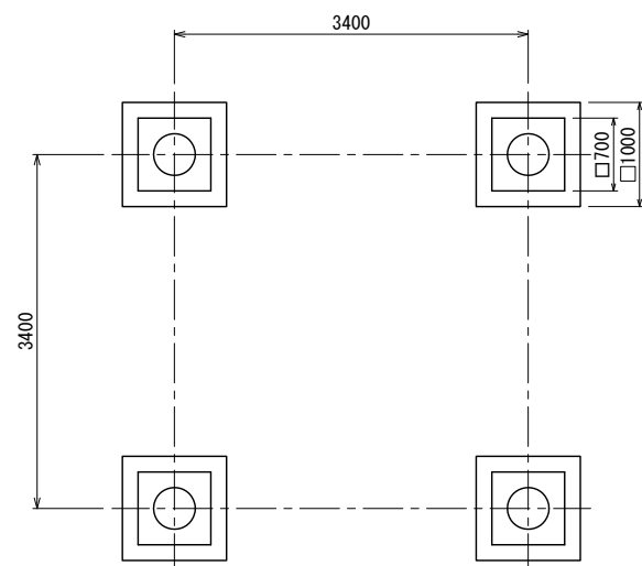
基礎伏図
