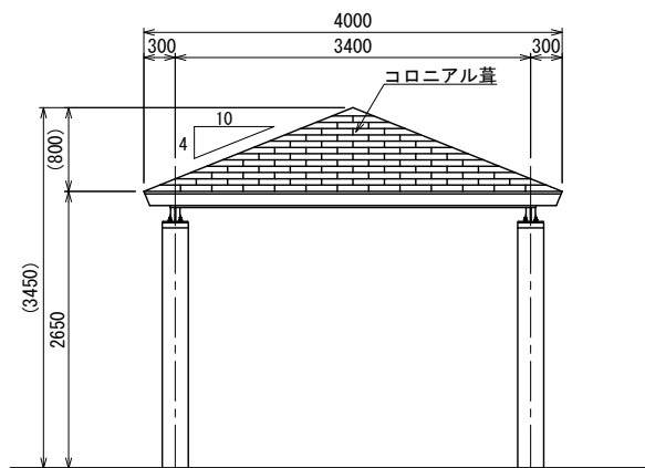
立面図
