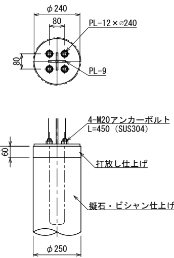
支柱上部取付詳細図 S=1:10 (A3 S=1:20)
